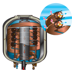
échangeur coaxial
