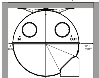
Contraintes d'installation en placard
